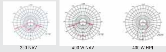
İŞIK DAĞILIM EĞRİLERİ - LIGHT DISTRIBUTION CURVES
